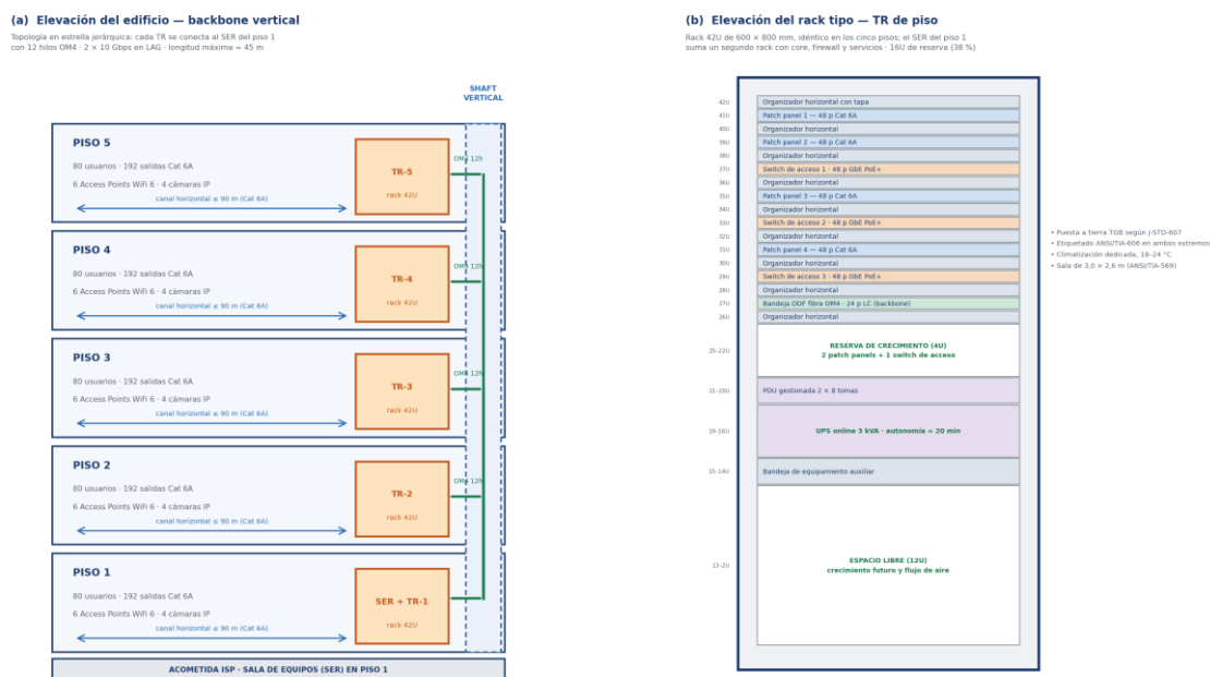
Figura 4. Elevación del edificio con el backbone vertical y elevación del rack tipo del cuarto de telecomunicaciones.
