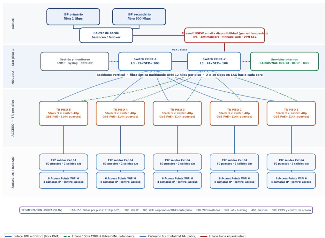
Figura 1. Topología lógica de la red. Arquitectura jerárquica de dos capas con núcleo colapsado redundante y segmentación por VLAN.
